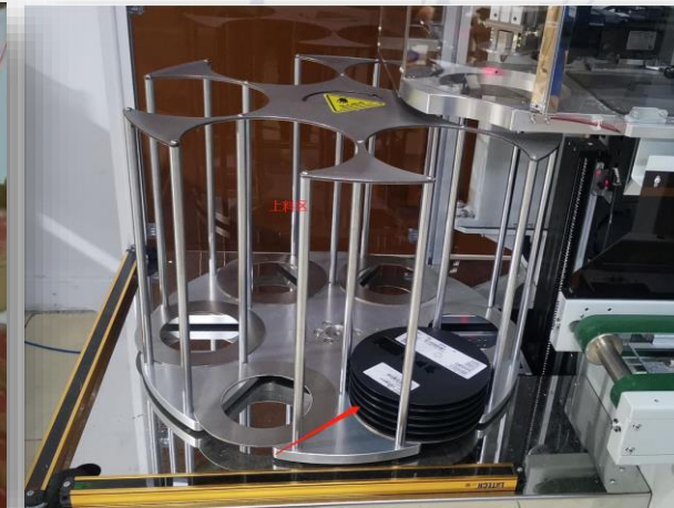
高效全能 工作效率约为1.6S/盘, 工作8小时可贴标、复核 12000-15000盘(约为 250箱)
